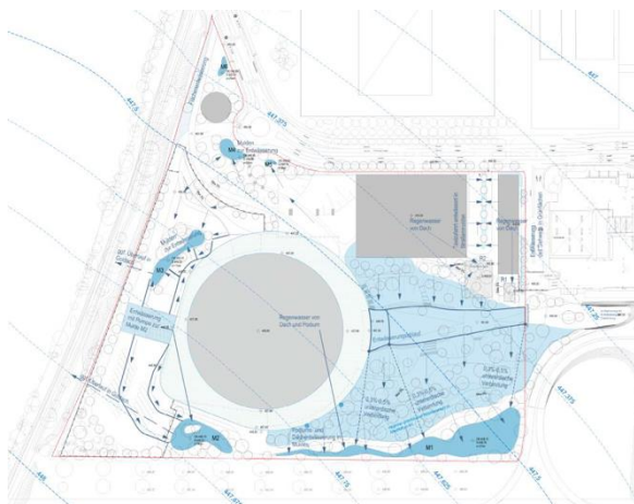
Abb.: Versickerungskonzept Vorhabensgebiet Latz und Partner, 2024
